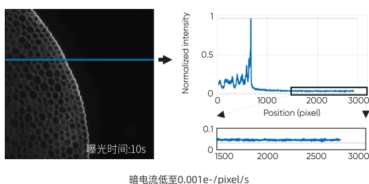
暗电流低至0.001e-/pixel/s
